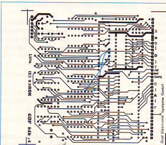
Abb. 7.9.25 Die Lötseite der Leiterplatte GDP64
