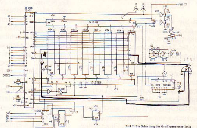
Bild 7. Die Schaltung des Grafikprozessor-Teils
